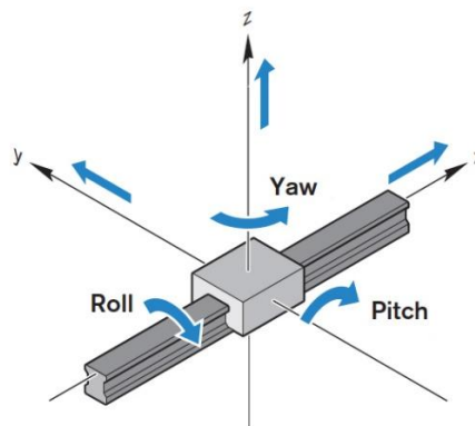
Gambar 8 Ilustrasi Sumbu Utama pada Koordinat Kartesius (Sumber: https://www.linearmotiontips.com/ )
